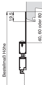
mit Winkelanbau
