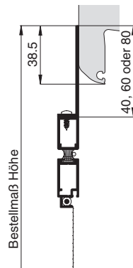
mit Winkelanbau
