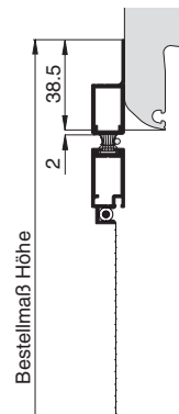
ohne Winkelanbau
