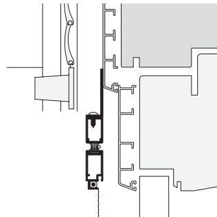
mit Winkelanbau
