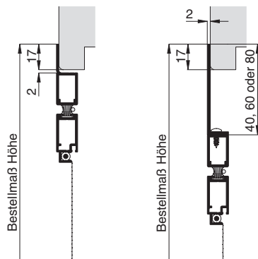
ohne Winkelanbau
